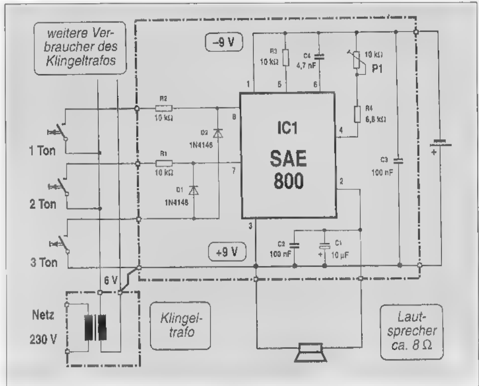
Figuur 1: Het schema van de 3-tonige gong.
